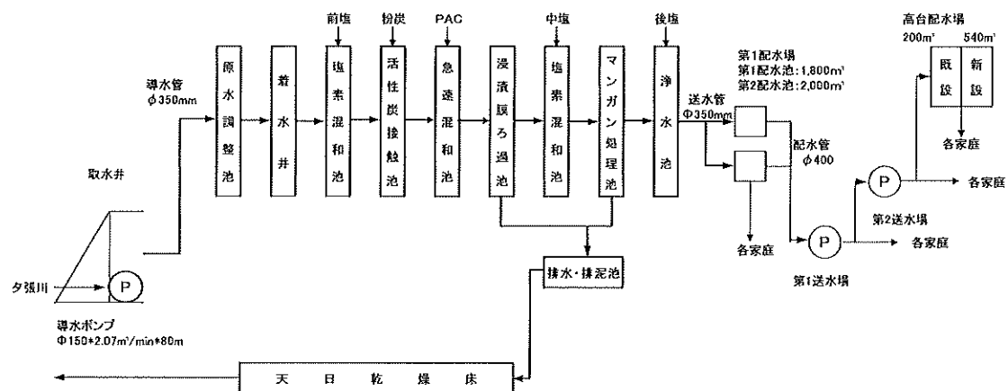
第 2 浄水場 フロー図
